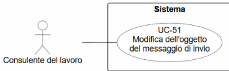
Figura 75: Diagramma del caso d'uso UC-51: Modifica dell'oggetto del messaggio di invio
