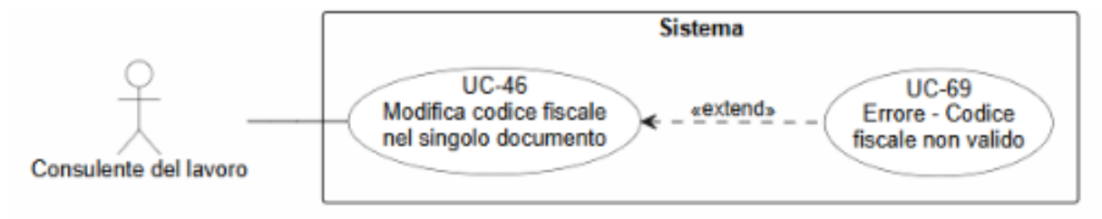
Figura 67: Diagramma del caso d'uso UC-46: Modifica codice fiscale nel singolo documento
