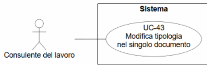
Figura 64: Diagramma del caso d'uso UC-43: Modifica tipologia nel singolo documento
