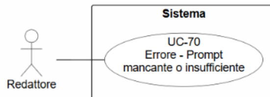
Figura 99: Diagramma del caso d'uso UC-70: Errore per prompt mancante o insufficiente
