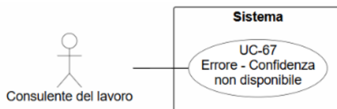
Figura 96: Diagramma del caso d'uso UC-67: Errore per confidenza non disponibile
