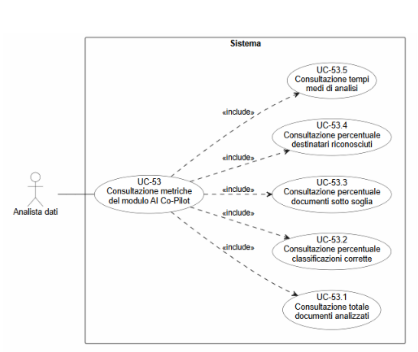
Figura 77: Diagramma del caso d'uso UC-53: Consultazione metriche del modulo AI Co-Pilot
