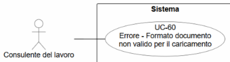
Figura 89: Diagramma del caso d'uso UC-60: Errore per formato documento non valido per il caricamento
