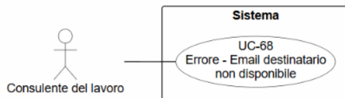
Figura 97: Diagramma del caso d'uso UC-68: Errore per email destinatario non disponibile
