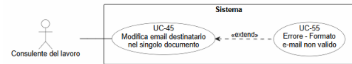
Figura 66: Diagramma del caso d'uso UC-45: Modifica email destinatario nel singolo documento
